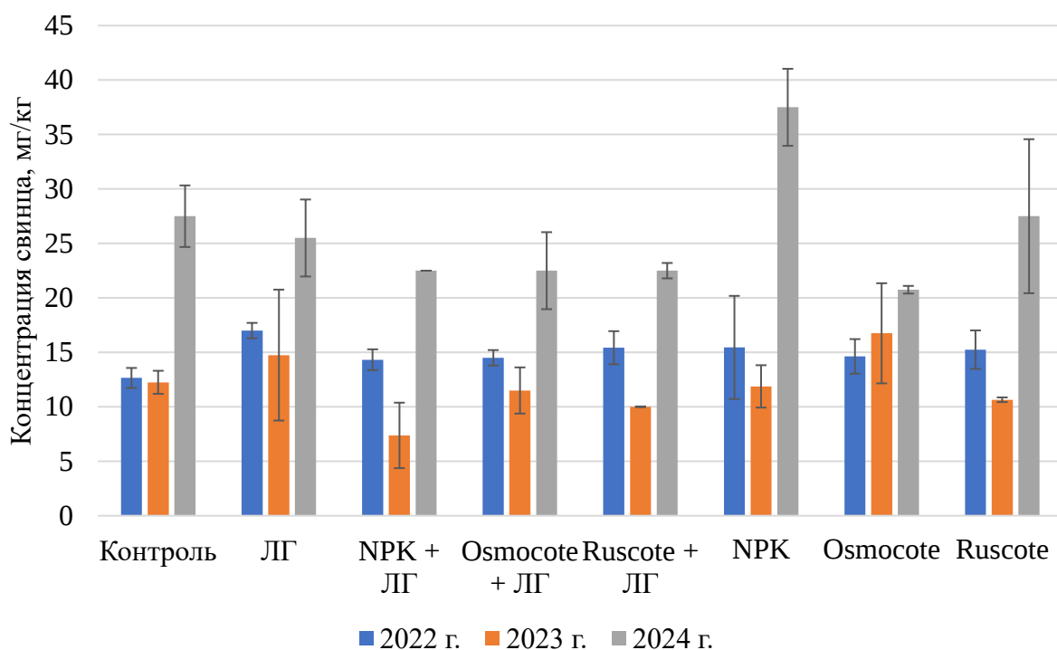
Рисунок 17. Содерание свинца (вытяжка - ААБ) в почвогрунте, мг/кг. Вертикальными линиями на графике отмечена ошибка опыта.
