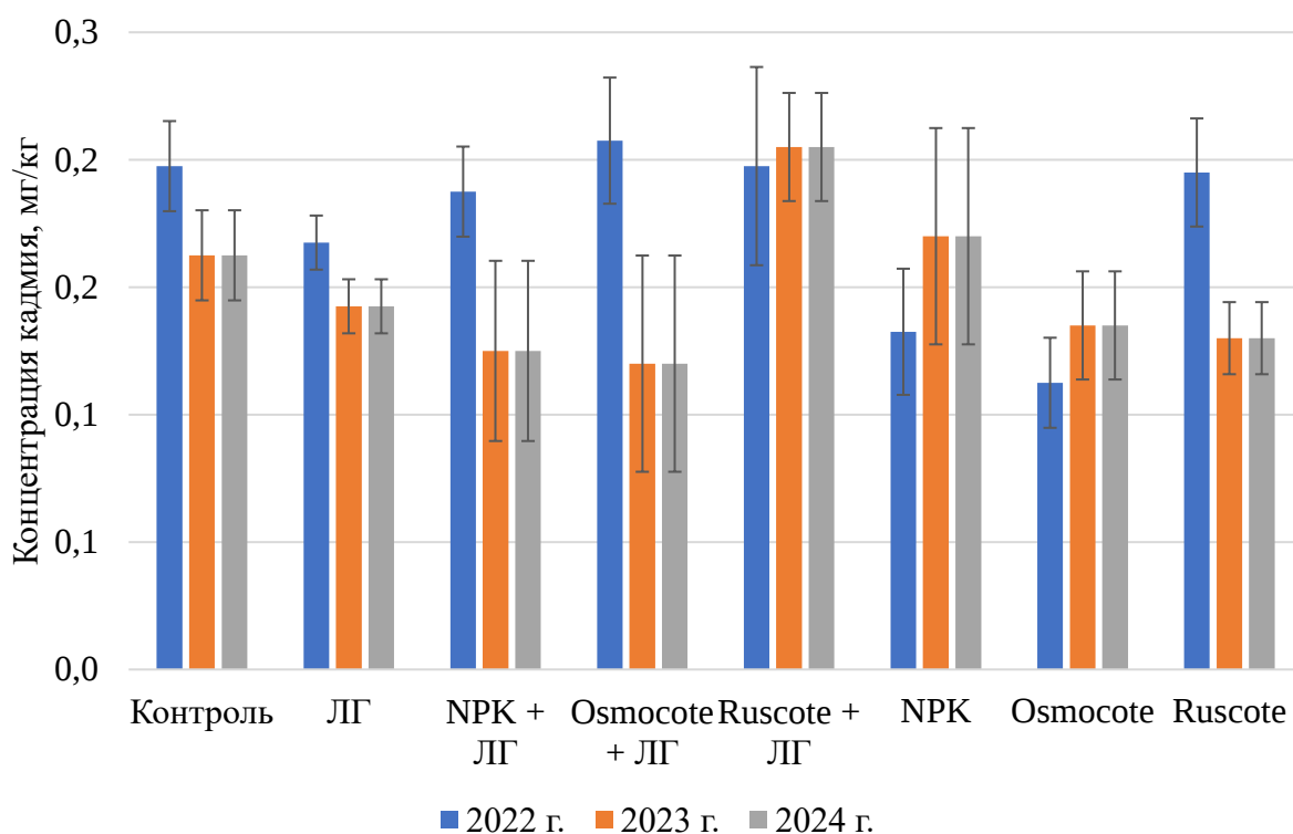
Рисунок 18. Содерание кадмия (вытяжка - ААБ) в почвогрунте, мг/кг. Вертикальными линиями на графике отмечена ошибка опыта.
