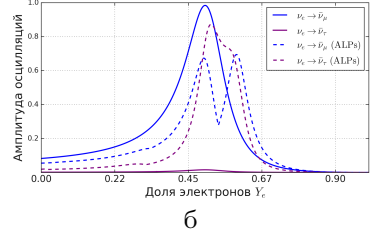
Рисунок 2 — Зависимость амплитуды осцилляций от доли электронов. Дираковская и майорановские CP-нарушающие фазы равны нулю, энергия нейтрино E_\nu = 10 МэВ; а – Осцилляции нейтрино-нейтрино; б – Осцилляции нейтрино-антинейтрино
