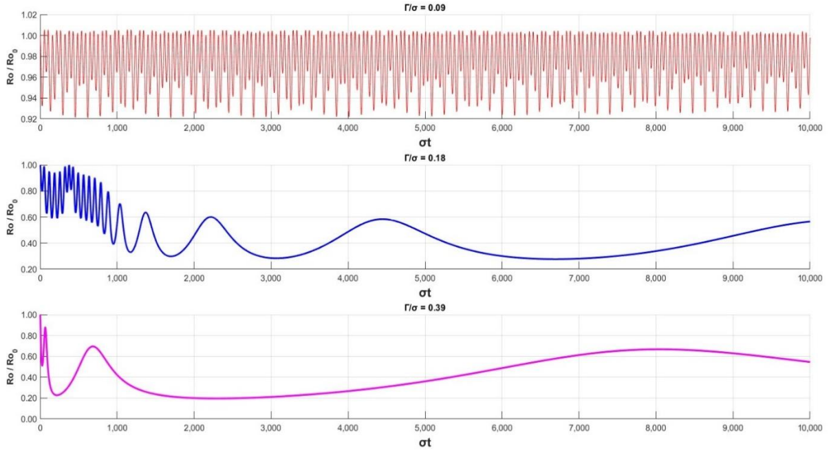
Рис.46. Зависимость относительного числа Россби \frac{R_O(\varepsilon, K)}{R_O(\varepsilon(0), K(0))} от безразмерного времени для трёх характерных режимов: режима выживания, конечного времени жизни и безграничного вытягивания (в порядке сверху вниз). Графики представлены при одинаковых начальных условиях: \varepsilon(0) = 1, K(0) = 0.25, \theta(0) = 0, \varphi(0) = 0, \psi(0) = 0 .
