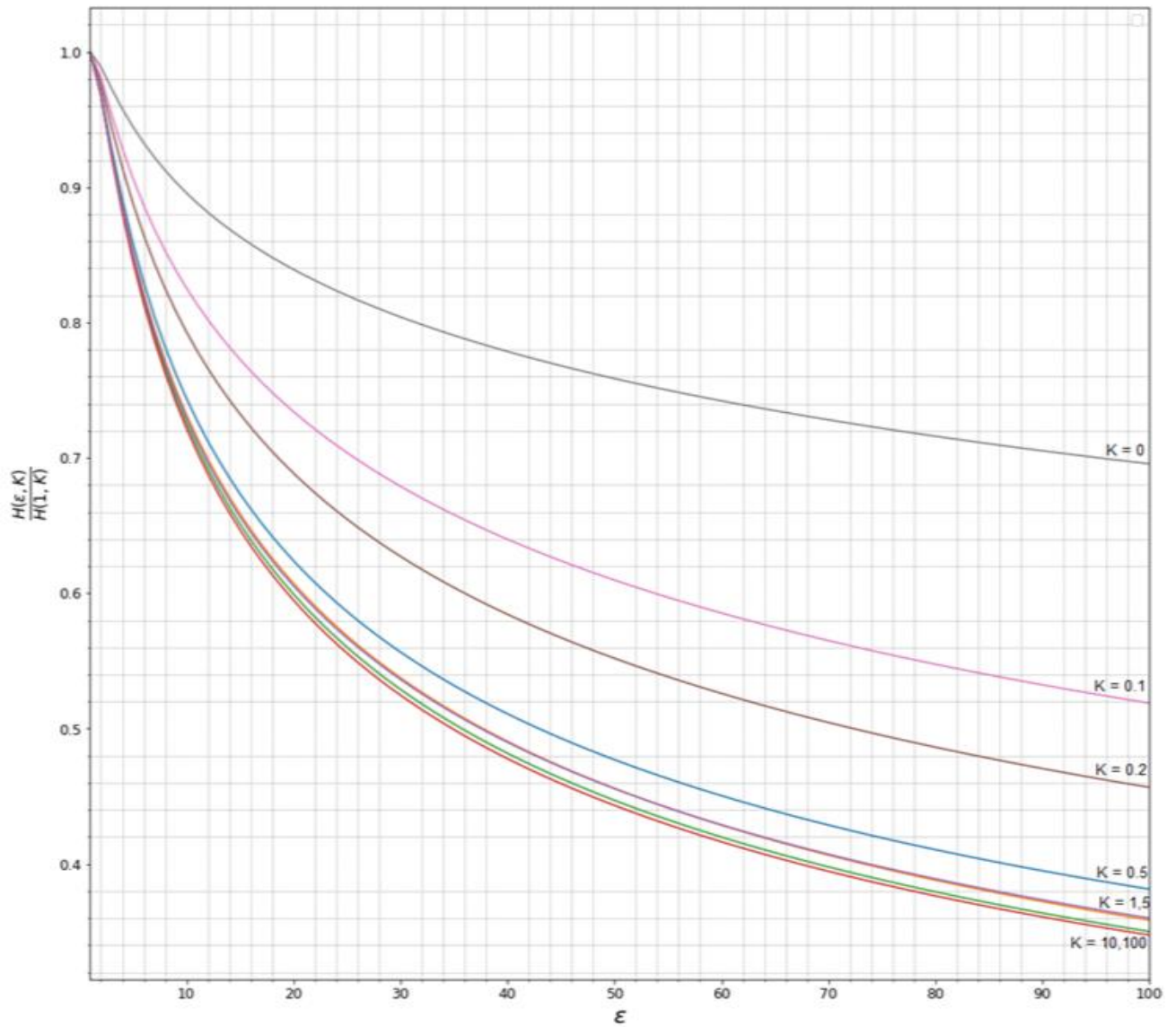
Рис.5. Зависимость нормированной полной механической энергии вихря \frac{H(\epsilon, K)}{H(1, K)} от безразмерного параметра вытягивания \epsilon при различных фиксированных значениях параметра сплюснутости K .
