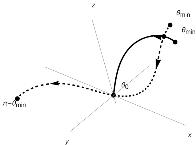
Рис. 4 Взаимное расположение аксоидов. Значение переменной -1 \leq h < 0
