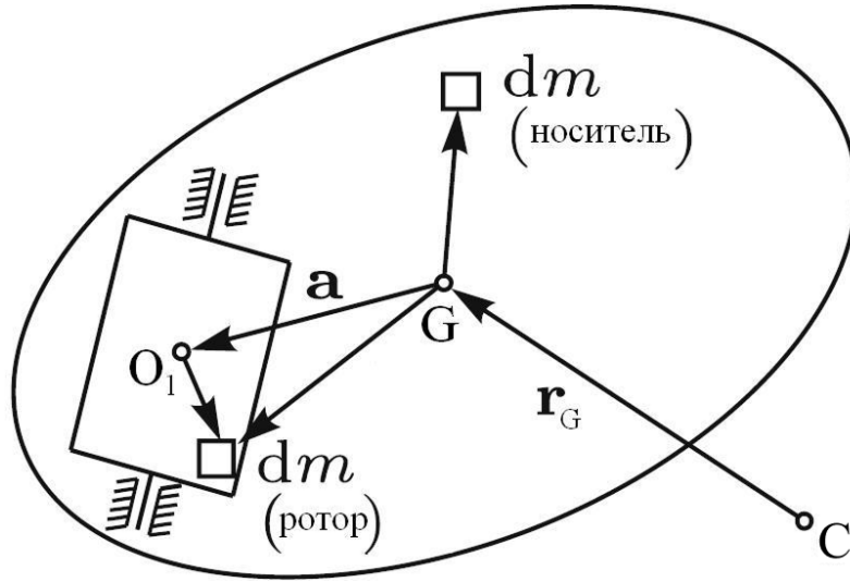
Рис. 1 Схематичный вид гиростата. Точкой C обозначена неподвижная точка пространства, r_G — радиус-вектор к центру масс системы
