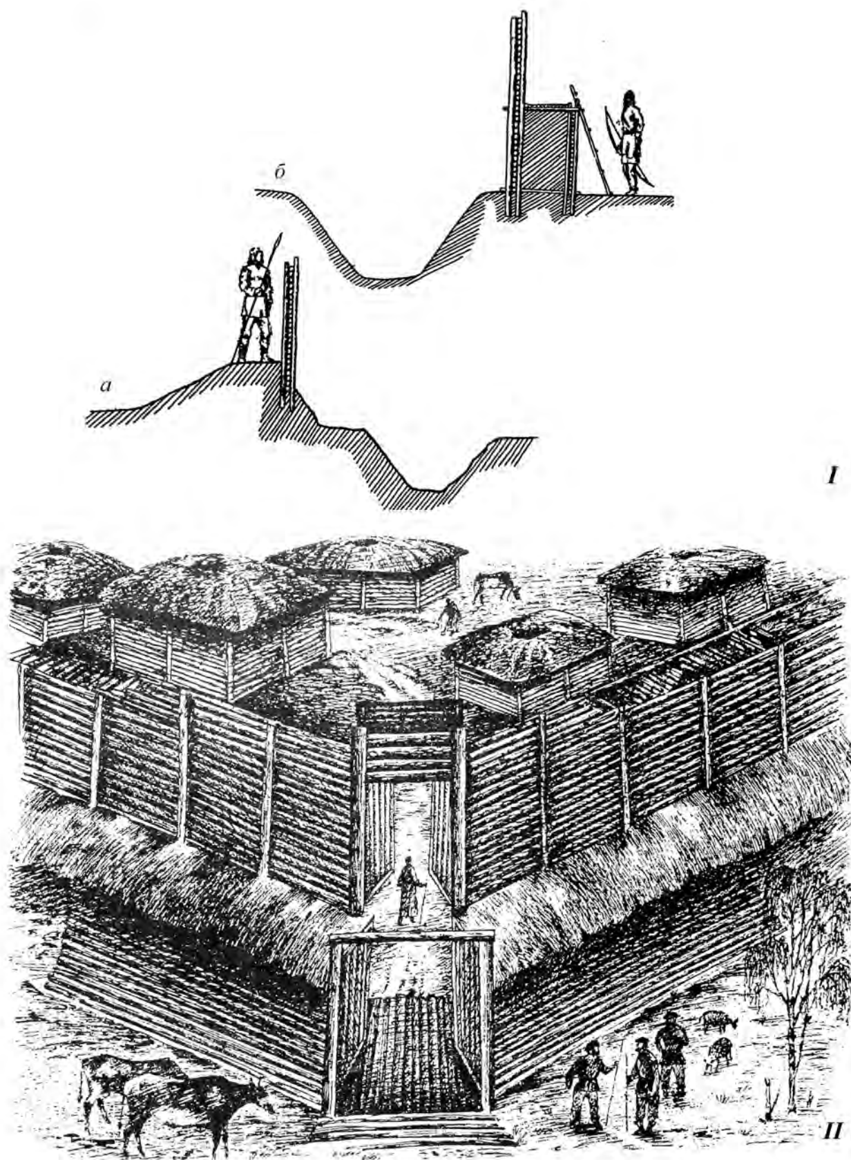
Рис. 121. Рафайловское городище. Реконструкции. I - однорядная защитная стена (a); двухрядная с забутовкой и настилом для стрелковой галереи (b); II - крепость раннего этапа (по Матвеева и др., 2005. Рис. 68, 69).
