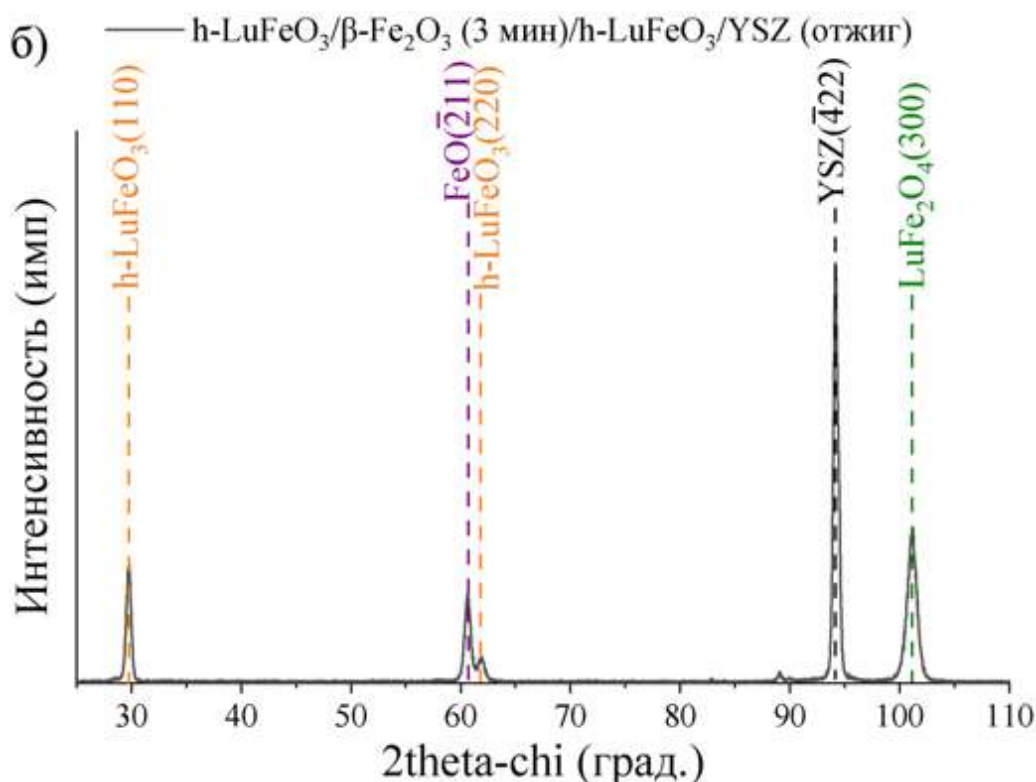
Рисунок 91. (а) \theta – 2\theta сканы образцов, полученных в процессе восстановительного отжига трехслойных гетероструктур h\text{-LuFeO}_3/\beta\text{-Fe}_2\text{O}_3/\text{YSZ} . (б) 2\theta – \chi – \phi скан образца, полученного при восстановлении гетероструктуры h\text{-LuFeO}_3/\beta\text{-Fe}_2\text{O}_3(3 \text{ мин})/h\text{-LuFeO}_3/\text{YSZ} .
