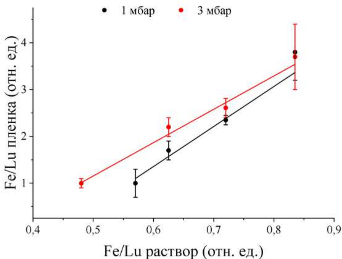
Рисунок 60. Зависимости соотношения Fe/Lu в плёнках « \text{LuFeO}_3 » от состава раствора прекурсоров при разных парциальных давлениях кислорода в реакторе MOCVD.
