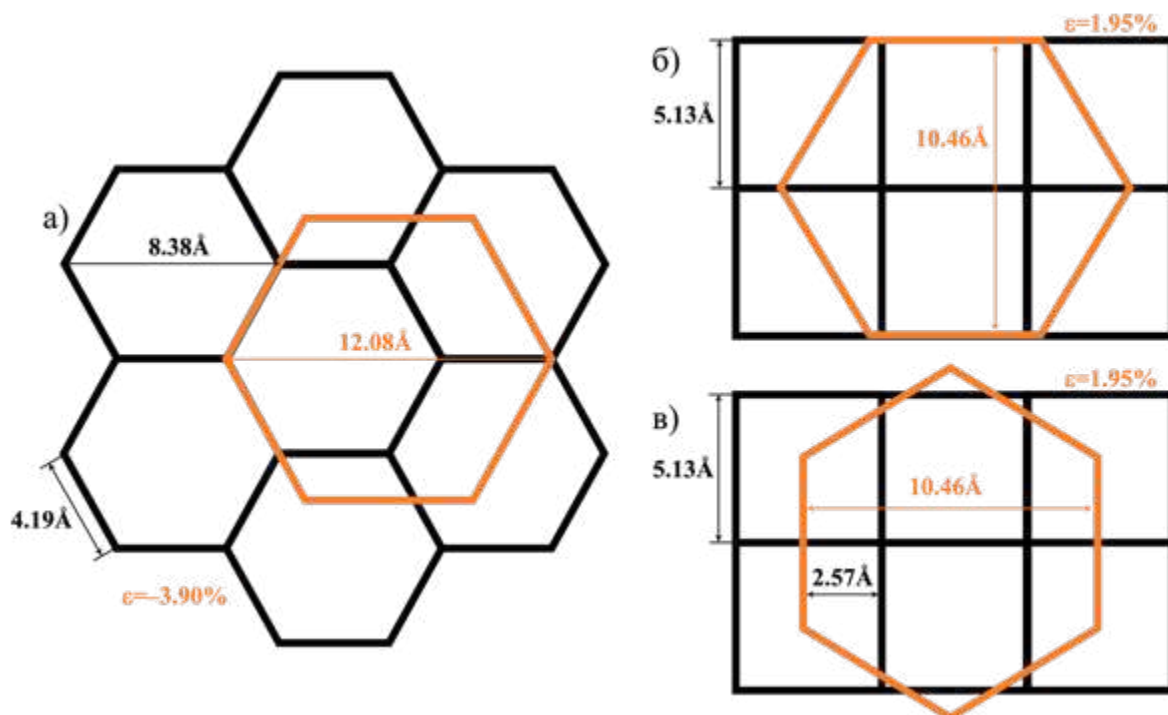
Рисунок 64. Варианты конфигураций интерфейсов (а) h\text{-LuFeO}_3(001) // \text{YSZ}(111) и (б), (в) h\text{-LuFeO}_3(001) // \text{YSZ}(001) с приведенными значениями рассогласования параметров элементарных ячеек ( \epsilon ) h\text{-LuFeO}_3 и YSZ. Оранжевым цветом отмечен контур ячейки h\text{-LuFeO}_3 , черным – YSZ.
