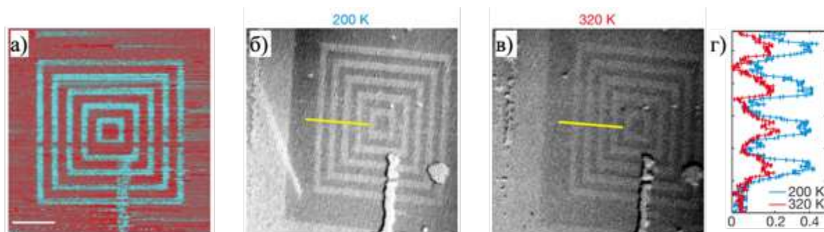
Рисунок 31. (а) PFM изображение сегнетоэлектрических доменов при 300 К. Домены были предварительно ориентированы вдоль оси c , голубым цветом обозначены домены с поляризацией, направленной вверх, красным – вниз. XMCD-PEEM изображения, полученные на Fe L_3 -крае при температуре (б) 200 К и (в) 320 К. (г) Сравнение дихроичных сигналов вдоль желтых линий на XMCD-PEEM изображениях [21].
