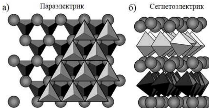
Рисунок 13. Тригональные бипирамиды изображают полиэдры \text{FeO}_5 , а сферы – катионы Lu. (а) Кристаллическая структура параэлектрического \text{h-LuFeO}_3 ( \text{P6}_3/\text{mmc} ) представляет собой последовательность наложенных друг на друга слоев из \text{FeO}_5 с зажатым между ними слоем Lu. (б) Вид сегнетоэлектрической фазы \text{h-LuFeO}_3 ( \text{P6}_3\text{cm} ) в направлении, перпендикулярном кристаллографической оси c .
