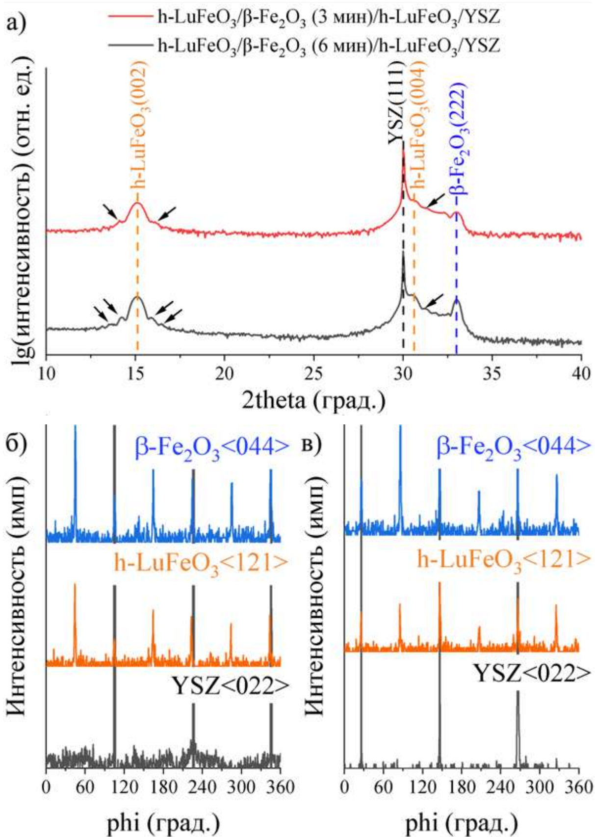
Рисунок 89. (а) \theta – 2\theta сканы трехслойных гетероструктур со слоями \beta\text{-Fe}_2\text{O}_3 , осаждаемыми в течение трех минут (красная линия) и шести минут (черная линия), на
