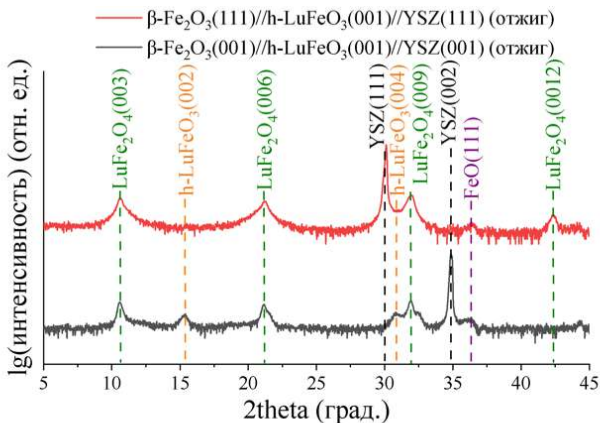
Рисунок 87. \theta – 2\theta сканы образцов, полученных в ходе восстановительного отжига тонкопленочных гетероструктур \beta\text{-Fe}_2\text{O}_3/\text{h-LuFeO}_3 на подложках YSZ(001) (черная линия) и YSZ(111) (красная линия).
