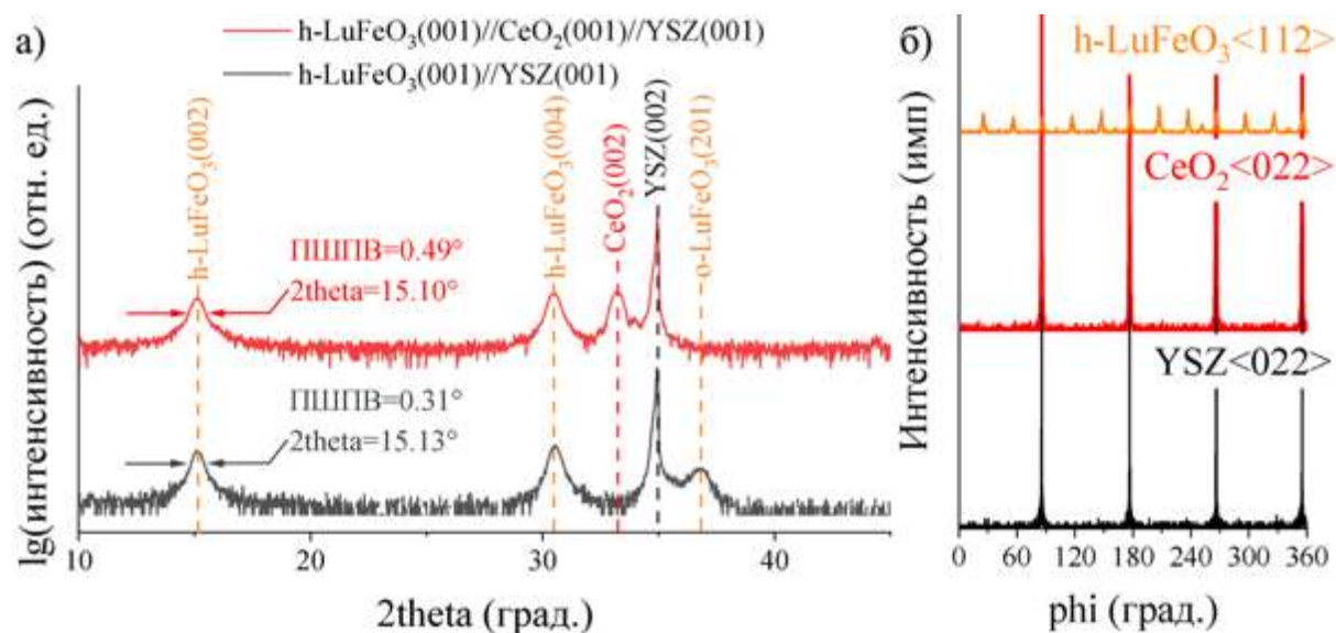
Рисунок 70. (а) \theta - 2\theta сканы плёнок h\text{-LuFeO}_3 на поверхности (001) флюоритных подложек YSZ (черная линия) и \text{CeO}_2/\text{YSZ} (красная линия). (б) \phi сканы кристаллографических направлений h\text{-LuFeO}_3\langle 112 \rangle , \text{CeO}_2\langle 022 \rangle и \text{YSZ}\langle 022 \rangle в гетероструктуре h\text{-LuFeO}_3(001) // \text{CeO}_2(001) // \text{YSZ}(001) .
