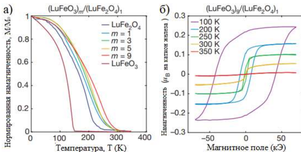
Рисунок 30. (а) M - T зависимости сверхструктур (\text{LuFeO}_3)_m/(\text{LuFe}_2\text{O}_4)_1 , охлажденных в магнитном поле 1 кЭ. M_0 – намагниченность при температуре 1.8 К. (б) Петли гистерезиса геткоструктуры в координатах M - H (намагниченность-индукция внешнего магнитного поля) при разных температурах [21].
