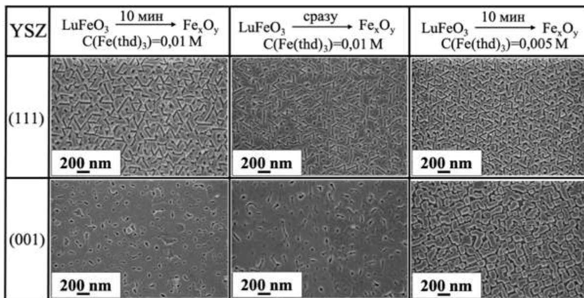
Рисунок 80. Микрофотографии гетероструктур, полученных на подложках YSZ(111)(верхний ряд) и YSZ(001) (нижний ряд). Условия осаждений слоя оксида железа изображены в верхнем ряду.
