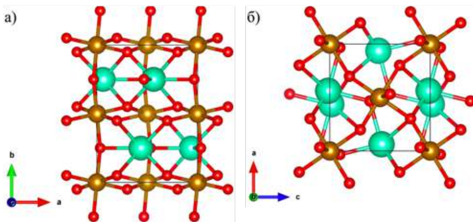
Рисунок 1. Вид элементарной ячейки \text{o-LuFeO}_3 вдоль кристаллографического направления (а) \langle 001 \rangle и (б) \langle 0k0 \rangle . Зеленые шарики обозначают позиции лутеция, золотые – железа, красные – кислорода [29].
