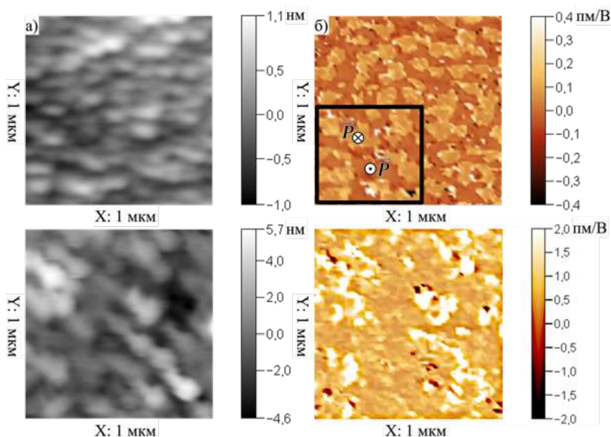
Рисунок 77. Снимки атомно-силовой микроскопии, демонстрирующие морфологию поверхности тонких пленок (а) h\text{-LuFeO}_3(001)/\text{YSZ}(111) и (в) h\text{-LuFeO}_3(001)/\text{YSZ}(001) . (б) и (г) представляют собой карты распределения сегнетоэлектрических доменов с тех же участков, с которых получены снимки АСМ. На вставке (б) отмечено соответствие направления вектора поляризации ( \vec{P} ) с цветом на изображении.
