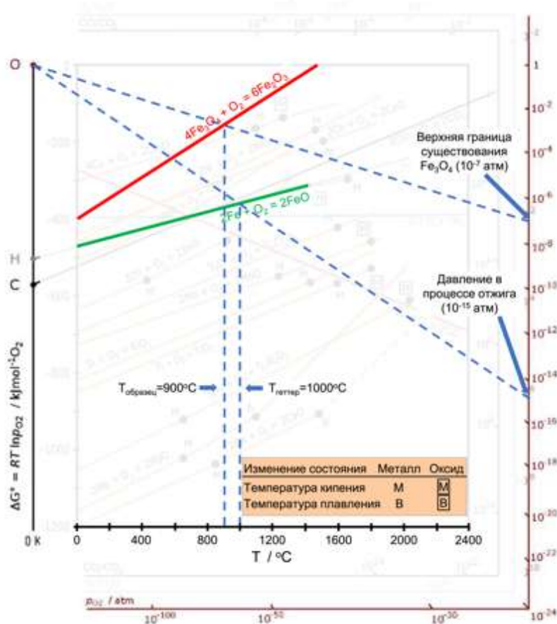
Рисунок 86. Диаграмма Эллингема [125] с обозначенными условиями восстановления гетероструктур \beta -Fe 2 O 3 /h-LuFeO 3 /YSZ.
