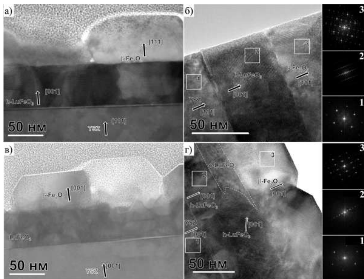
Рисунок 81. Микрофотографии поперечных срезов гетероструктур (а), (б) \beta\text{-Fe}_2\text{O}_3(111)/h\text{-LuFeO}_3(001)/\text{YSZ}(111) и (в), (г) \beta\text{-Fe}_2\text{O}_3(001)/h\text{-LuFeO}_3(001)/\text{YSZ}(001) . На вставках приведены Фурье-преобразования отмеченных участков изображений, индцированием которых и был определен фазовый состав исследуемых гетероструктур.
