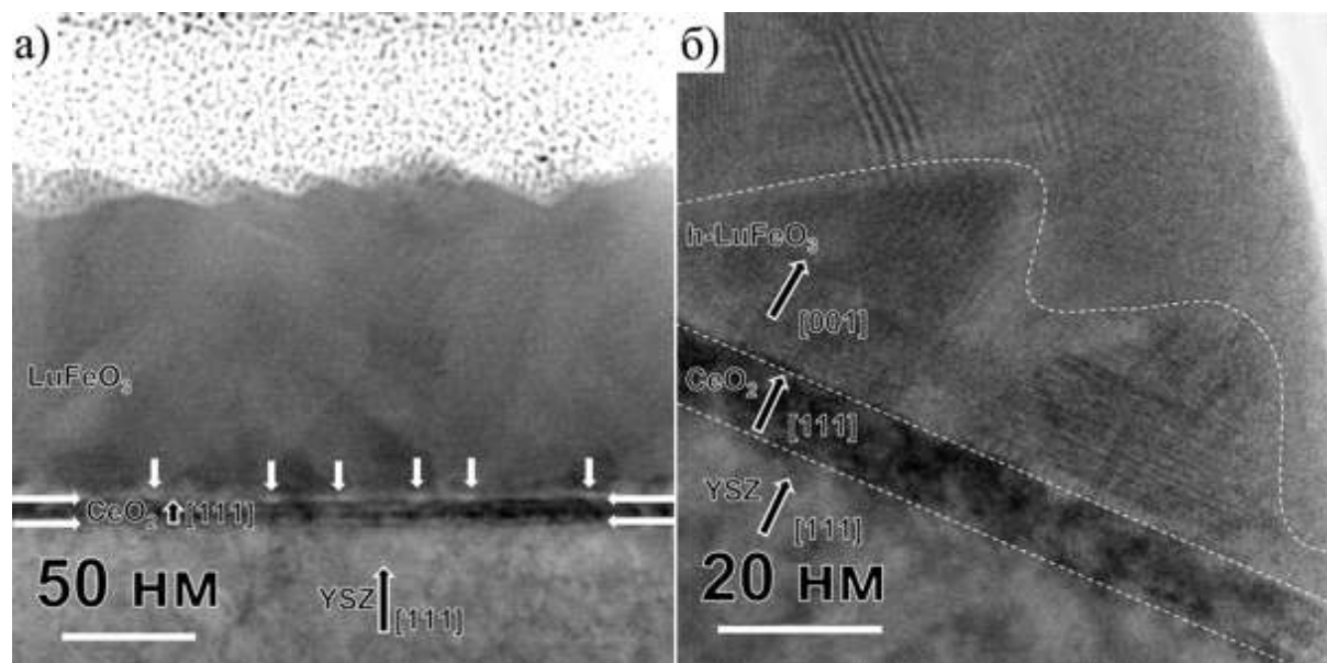
Рисунок 72. Микрофотографии поперечного среза гетероструктуры \text{h-LuFeO}_3(001)//\text{CeO}_2(111)//\text{YSZ}(111) . Белыми стрелками на (а) отмечены дислокации несоответствия на интерфейсе \text{h-LuFeO}_3(001)//\text{CeO}_2(111) .
