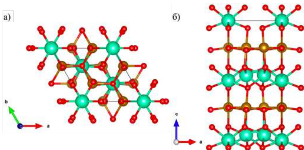
Рисунок 2. Вид элементарной ячейки \text{h-LuFeO}_3 вдоль кристаллографического направления (а) \langle 00l \rangle и (б) \langle 0k0 \rangle . Зеленые шарики обозначают позиции лутеция, золотые – железа, красные – кислорода [29].
