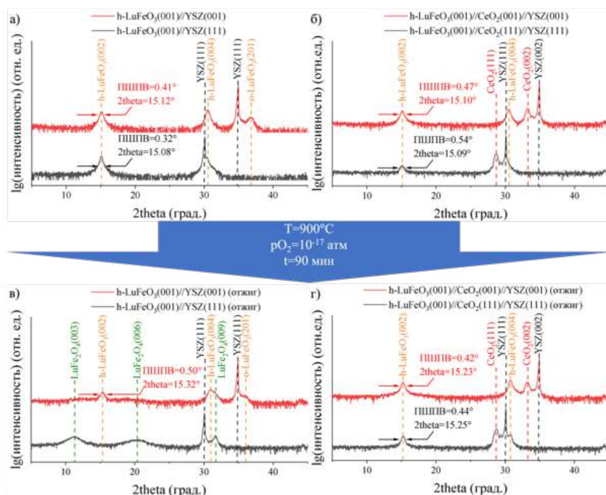
Рисунок 75. \theta – 2\theta сканы плёнок h\text{-LuFeO}_3 на поверхностях (111) (черная линия) и (001) (красная линия) (а) YSZ и (б) \text{CeO}_2 до восстановительного отжига, и (в) и (г) – после отжига.
