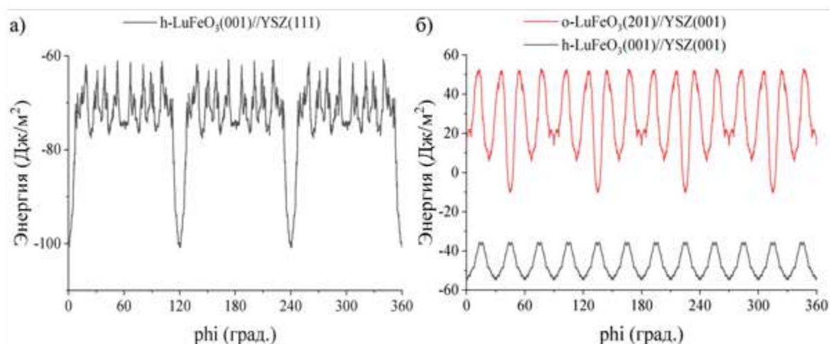
Рисунок 65. Рассчитанные энергетические профили интерфейсов (а) \text{h-LuFeO}_3(001)/\text{YSZ}(111) , (б красная линия) \text{o-LuFeO}_3(201)/\text{YSZ}(100) и (б черная линия) \text{h-LuFeO}_3(001)/\text{YSZ}(100) .
