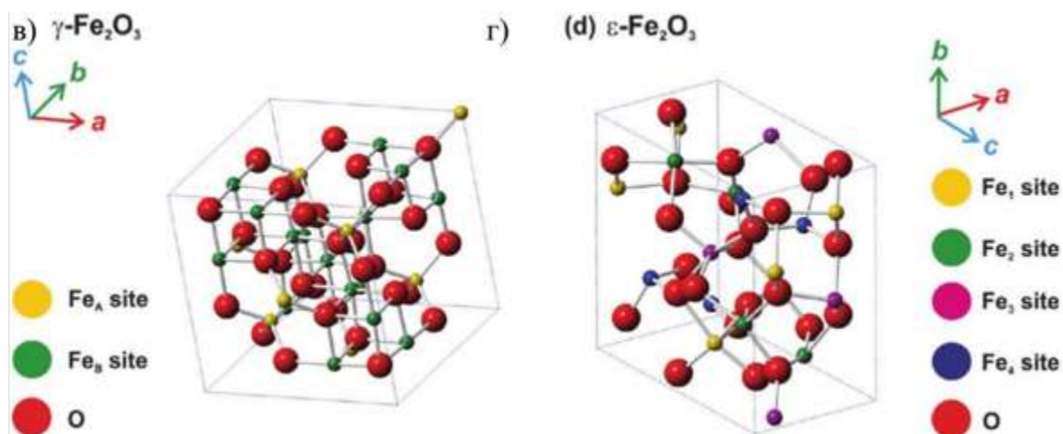
Рисунок 6. Элементарные ячейки четырех полиморфных модификаций \text{Fe}_2\text{O}_3 : (а) \alpha\text{-Fe}_2\text{O}_3 , (б) \beta\text{-Fe}_2\text{O}_3 , (в) \gamma\text{-Fe}_2\text{O}_3 и (г) \varepsilon\text{-Fe}_2\text{O}_3 [38].
