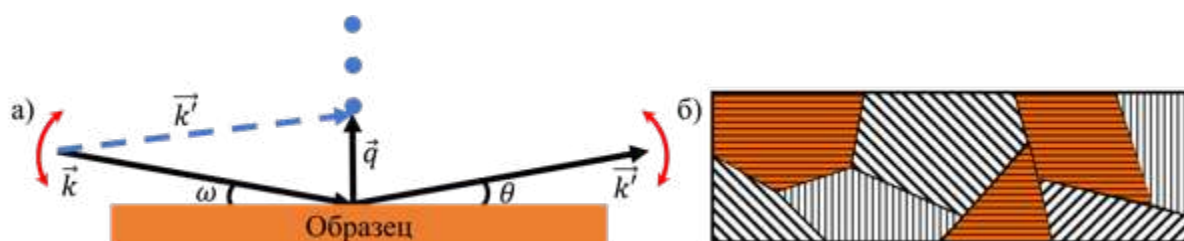
Рисунок 42. (а) Направления волновых векторов первичного, вторичного пучков и дифракционного вектора; красные стрелки отмечают движения осей дифрактометра при \theta - 2\theta сканировании. (б) Кристаллиты, плоскости которых находятся в отражающем положении при \theta - 2\theta сканировании.
