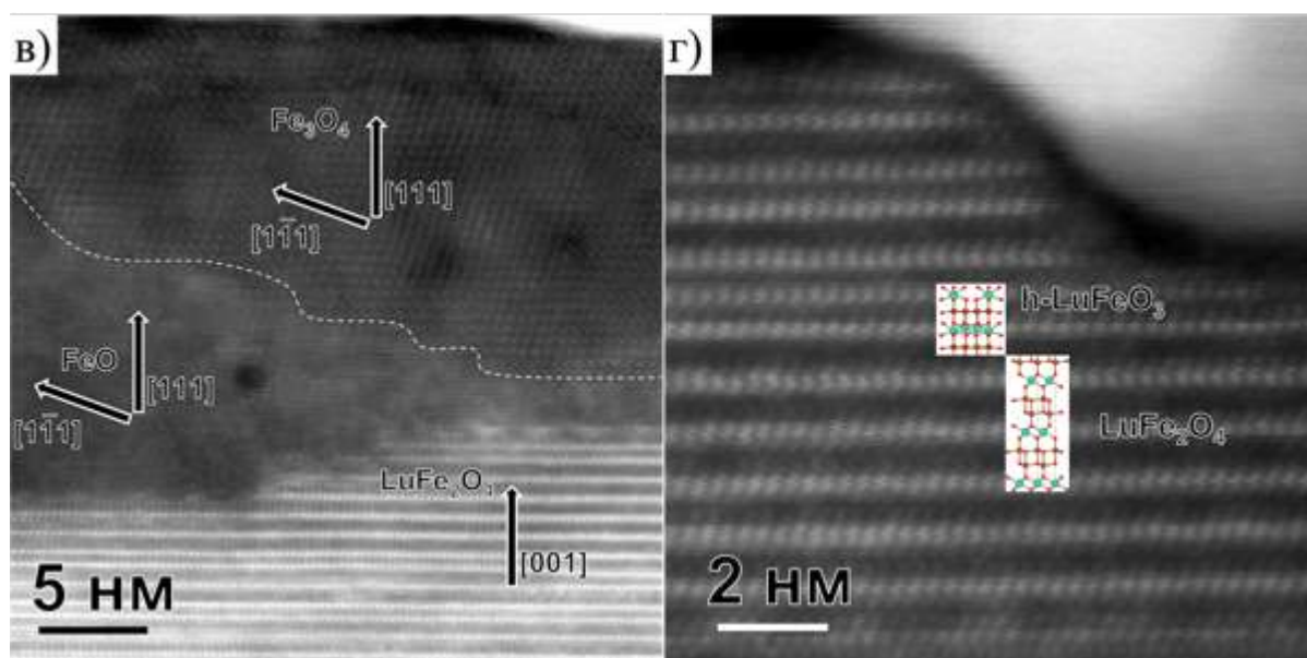
Рисунок 93. Микрофотографии поперечного среза восстановленной гетероструктуры \text{h-LuFeO}_3/\beta\text{-Fe}_2\text{O}_3(3 \text{ мин})/\text{h-LuFeO}_3/\text{YSZ} . (б), (в) Увеличенные микрофотографии, демонстрирующие границу между островком \text{FeO}/\text{Fe}_3\text{O}_4 и матрицей \text{LuFe}_2\text{O}_4/\text{h-LuFeO}_3 . (г) Микрофотография, демонстрирующая сросшиеся через слой \text{FeO} фазы \text{h-LuFeO}_3 и \text{LuFe}_2\text{O}_4 .
