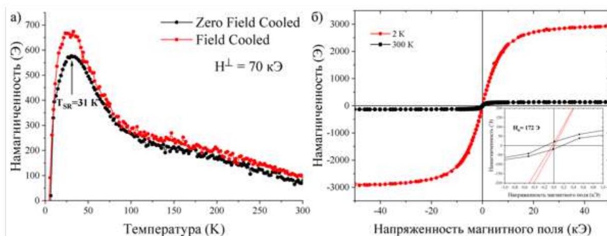
Рисунок 94. (а) Зависимость намагниченности образца \beta -Fe 2 O 3 (111)// h -LuFeO 3 (001)//YSZ(111) от температуры, зафиксированная в режимах FC (красная линия) и ZFC (черная линия). (б) Зависимость намагниченности этого же образца от напряженности внешнего магнитного поля при 300 К (черная линия) и 2 К (красная линия).
