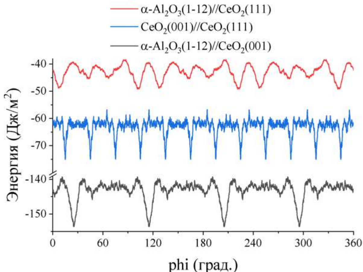
Рисунок 50. Энергетические профили интерфейсов \alpha\text{-Al}_2\text{O}_3(1\text{-}12)//\text{CeO}_2(111) (красная линия), \text{CeO}_2(111)//\text{CeO}_2(001) (синяя линия) и \alpha\text{-Al}_2\text{O}_3(1\text{-}12)//\text{CeO}_2(001) (черная линия).
