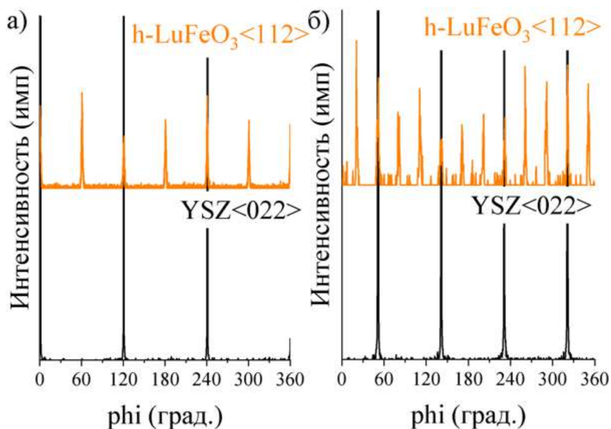
Рисунок 63. \phi сканы кристаллографических направлений h\text{-LuFeO}_3\langle 112 \rangle и \text{YSZ}\langle 022 \rangle показывающие взаимную ориентацию в плоскости ячеек h\text{-LuFeO}_3 и YSZ в пленках (а) h\text{-LuFeO}_3(001)//\text{YSZ}(111) и (б) h\text{-LuFeO}_3(001)//\text{YSZ}(001) .
