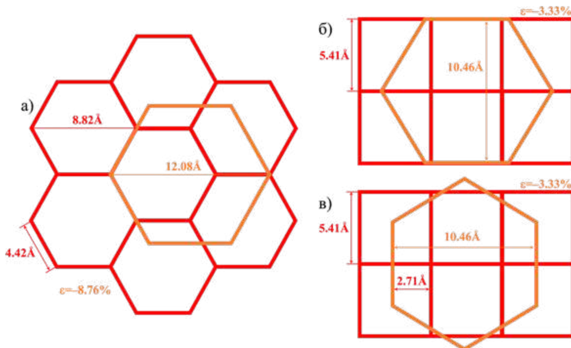
Рисунок 74. Варианты конфигураций интерфейсов (а) \text{h-LuFeO}_3(001)//\text{CeO}_2(111) и (б), (в) \text{h-LuFeO}_3(001)//\text{CeO}_2(001) с приведенными значениями рассогласования параметров
