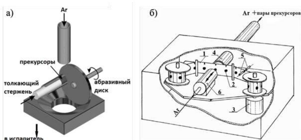
Рисунок 36. (а) Схема дозирующего устройства абразивного типа с использованием твёрдых прекурсоров [10]. (б) Схема питания с ленточным испарителем. 1 – стеклолента, 2 – высушенная капля прекурсора, 3 – двигатель, 4 – реакторная трубка, 5 – оптический сенсор, 6 – нагреватель [97].
