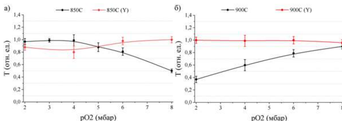
Рисунок 52. Зависимость текстурного коэффициента ориентации (001) CeO_2 от p(O_2) и содержания легирующего компонента (оксида иттрия) при температуре осаждения (а) 850°C и (б) 900°C.
