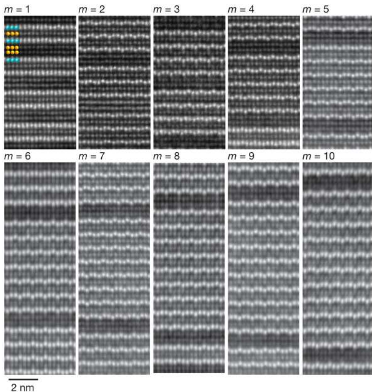
Рисунок 29. Результаты HRTEM гетероструктур (\text{LuFeO}_3)_m/(\text{LuFe}_2\text{O}_4)_1 , где m=1\div 10 [21].
