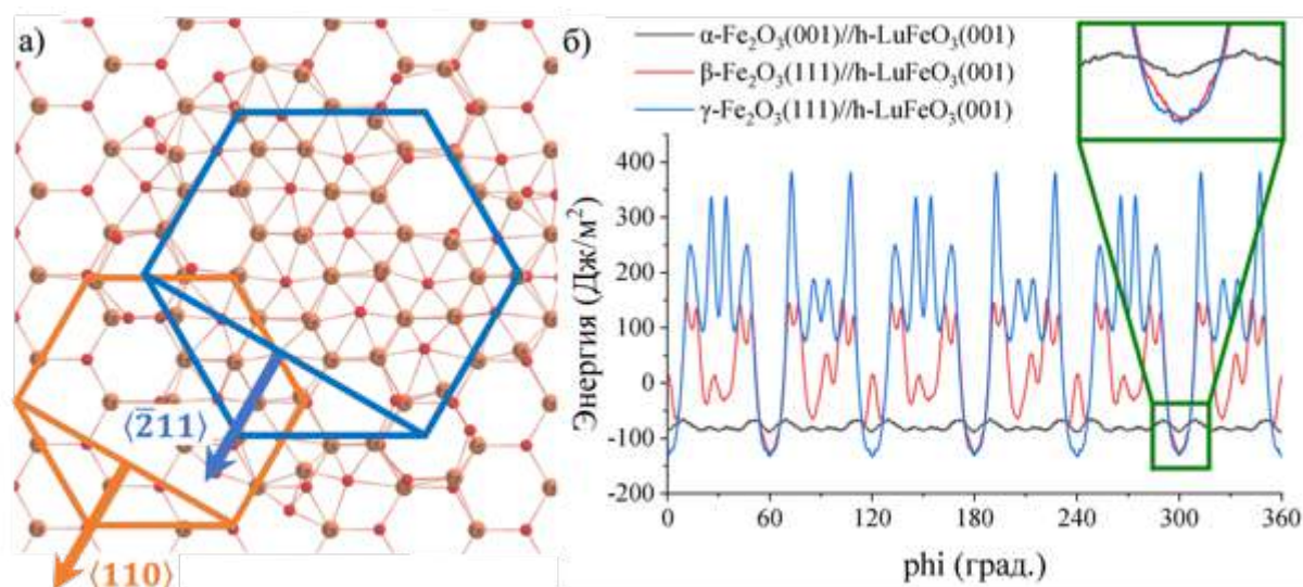
Рисунок 84. (а) Атомная конфигурация интерфейса h-LuFeO 3 (001)// \beta -Fe 2 O 3 (111). (б) Рассчитанные энергетические профили интерфейсов h-LuFeO 3 (001)// \alpha -Fe 2 O 3 (001) (черная линия), h-LuFeO 3 (001)// \beta -Fe 2 O 3 (111) (красная линия), h-LuFeO 3 (001)// \gamma -Fe 2 O 3 (111) (синяя линия).
