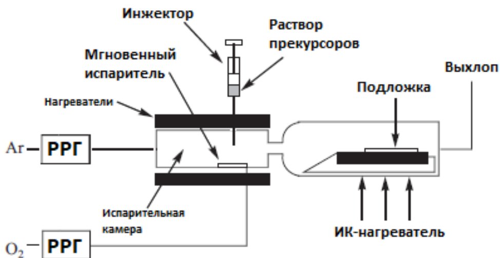
Рисунок 35. Схема МOCVD установки с модулем жидкостной инъекции для подачи прекурсоров [95].
