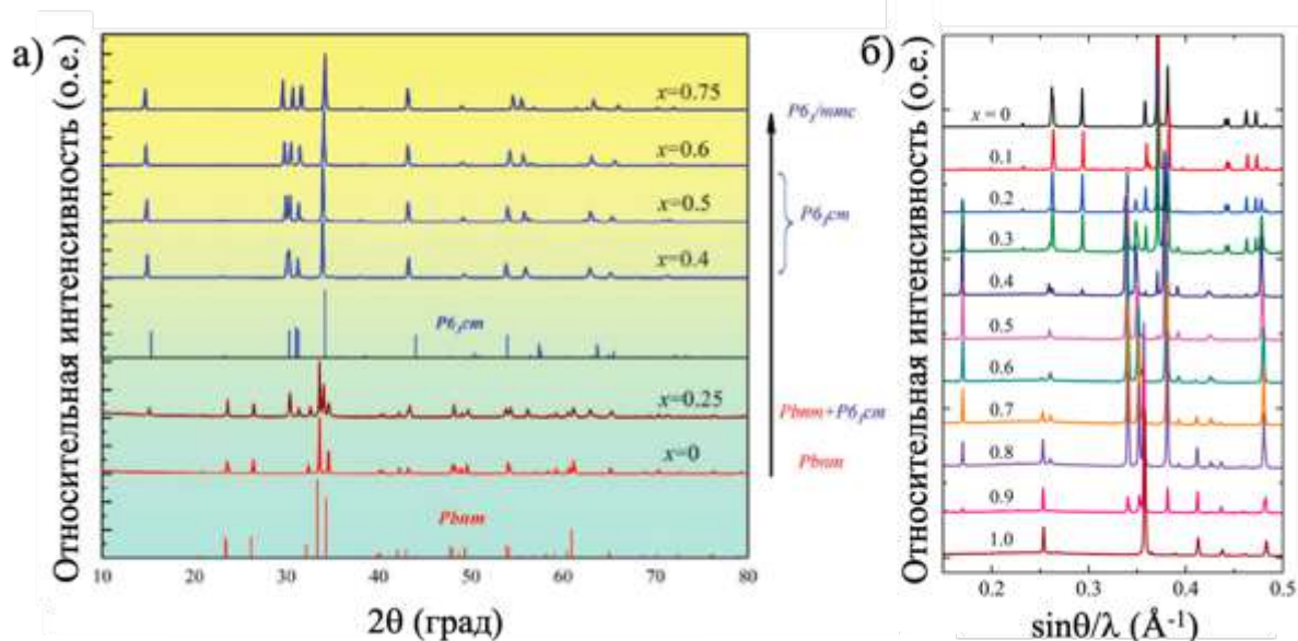
Рисунок 19. Дифрактограммы порошков \text{Lu}_{1-x}\text{In}_x\text{FeO}_3 ( x=0 - 0.75 ), \lambda=1.54059 \text{ \AA} (а) [86] и \text{Lu}_{1-x}\text{Sc}_x\text{FeO}_3 ( x=0 - 1 ), \lambda=0.49608 \text{ \AA} (б) [87].
