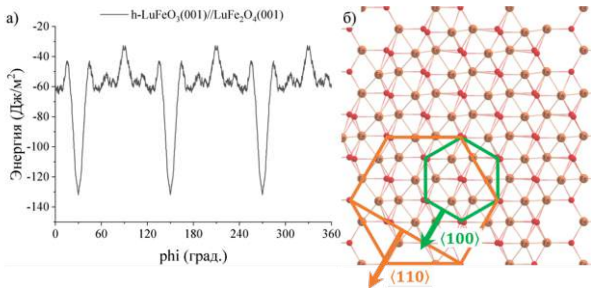
Рисунок 92. (а) Энергетический профиль, рассчитанный для интерфейса h\text{-LuFeO}_3(001)/\text{LuFe}_2\text{O}_4(001) и (б) атомная конфигурация данного интерфейса, установленная в результате расчета.
