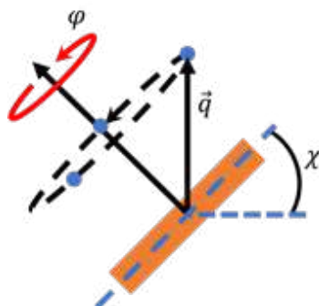
Рисунок 44. Схема с направление осей \phi и \chi при \phi сканировании, в данном случае изображен вид образца в плоскости «первичный пучок – вторичный пучок».
