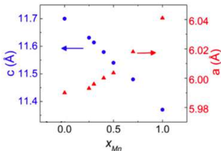
Рисунок 21. Зависимость параметров элементарной ячейки \text{LuFe}_{1-x}\text{Mn}_x\text{O}_3 от степени замещения железа на марганец [12].
