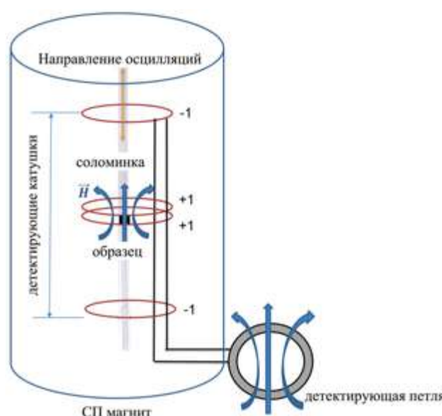
Рисунок 46. Иллюстрация устройства СКВИД [35].
