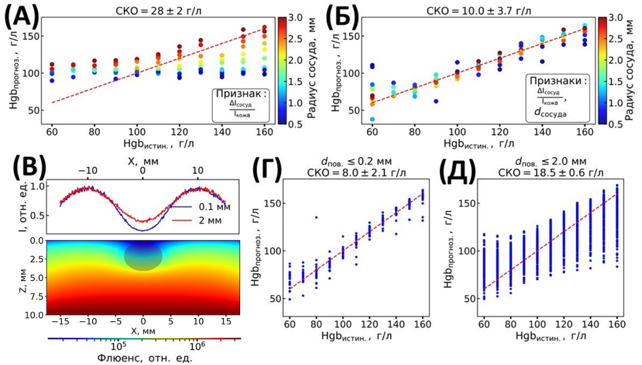
Рисунок 11. (А) Сопоставление Hgb прогноз. и Hgb истин. для моделей, использующих только относительный оптический контраст сосуда \Delta I_{\text{сосуд}}/I_{\text{ткань}} . (Б) Повышение точности модели при дополнительном учёте ширины сосуда d_{\text{сосуд}} . (В) Влияние глубины залегания сосуда на снижение контраста оптического сигнала. (Г, Д) Сравнение ошибок определения Hgb при малой глубине сосуда (0.2 мм) и глубокой локализации (1 мм)
