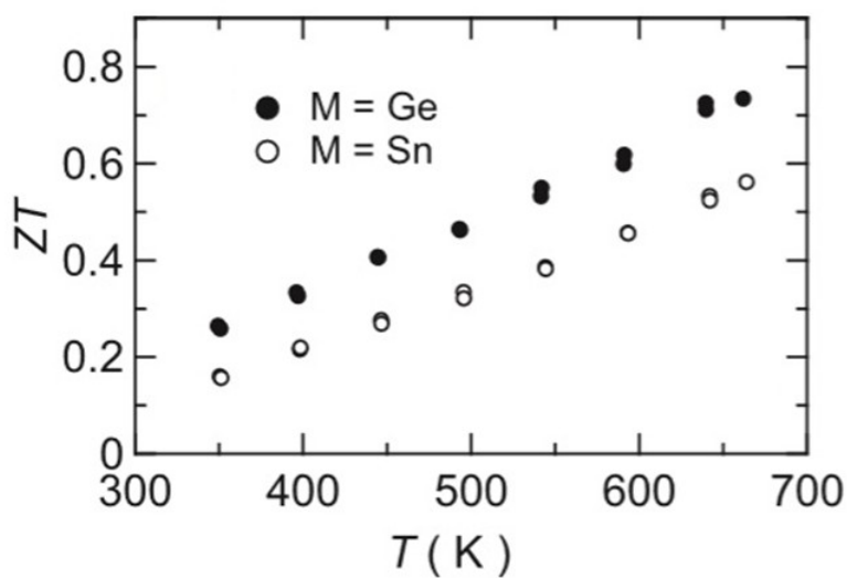
Рисунок 14. Температурная зависимость термоэлектрической добротности колюзитов \text{Cu}_{26}\text{V}_2\text{M}_6\text{S}_{32} (M = Sn, Ge) [82].
