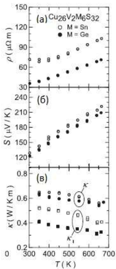
Рисунок 13. Температурная зависимость электрического сопротивления (а), коэффициента Зеебека (б) и теплопроводности (в) \text{Cu}_{26}\text{V}_2\text{M}_6\text{S}_{32} (M = Sn, Ge)[82].
