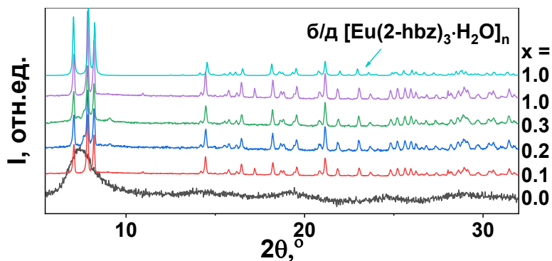
Рисунок 2 – Дифрактограммы \text{Eu}_x\text{Tb}_{1-x}(\text{2-hbz})_3(\text{H}_2\text{O})
