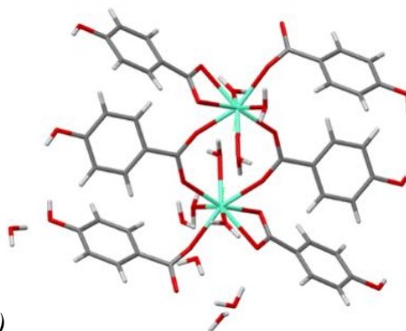
Рисунок 3 – (а-б) Структуры КС, на вставке – порошок \text{Eu}_{0.2}\text{Tb}_{0.8}(\text{3-hbz})_3(\text{H}_2\text{O})_4 и кристалл
