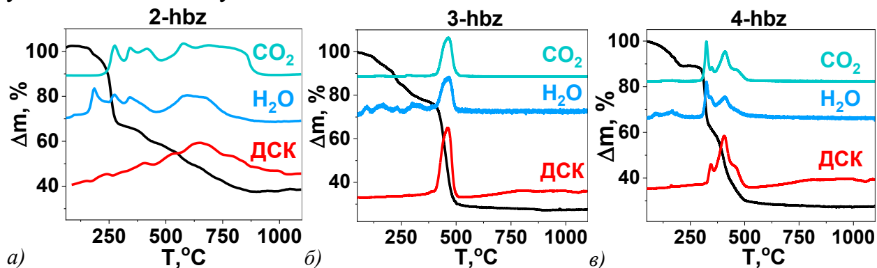
Рисунок 4 – (а-в) ТГА Eu_{0.2}Tb_{0.8}(hbz)_3(H_2O)_n
