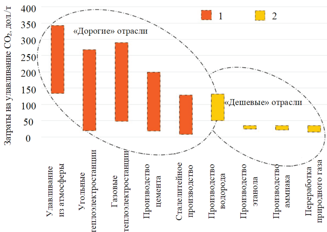
Рисунок 3 – Стоимость улавливания CO 2 (концентрация газа: 1 – низкая; 2 – высокая) Источник: 19
