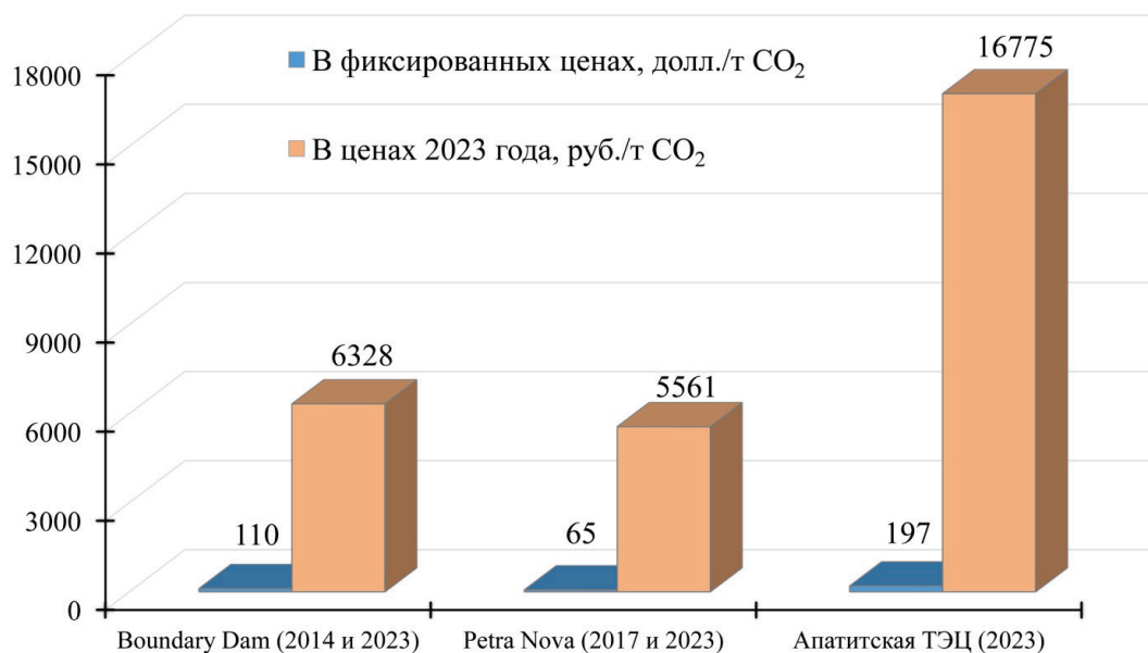
Рисунок 5 – Стоимость улавливания CO 2 на Апатитской ТЭЦ и объектах-аналогах Источник: составлено автором.
