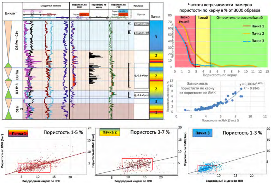
Рисунок 8. Характерные зависимости определений пористости пород по керну и по геофизическим методам исследований скважин для выделенных пачек пород.
