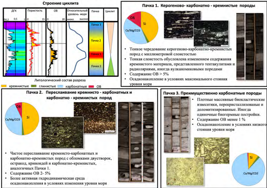
Рисунок 7. Строение циклита и характеристика пачек, слагающих циклит
