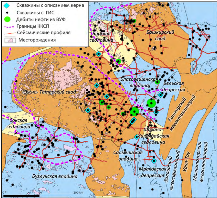
Рисунок 1. Структурные элементы и фактический материал района работ
