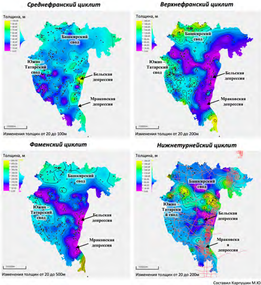
Рисунок 6. Распределение толщин франко-турнейского комплекса по цикллитам. Минимальные мощности фиксируют положение внутривпадинной впадины в среднефранское, позднефранское, фаменское и турнейское время.
