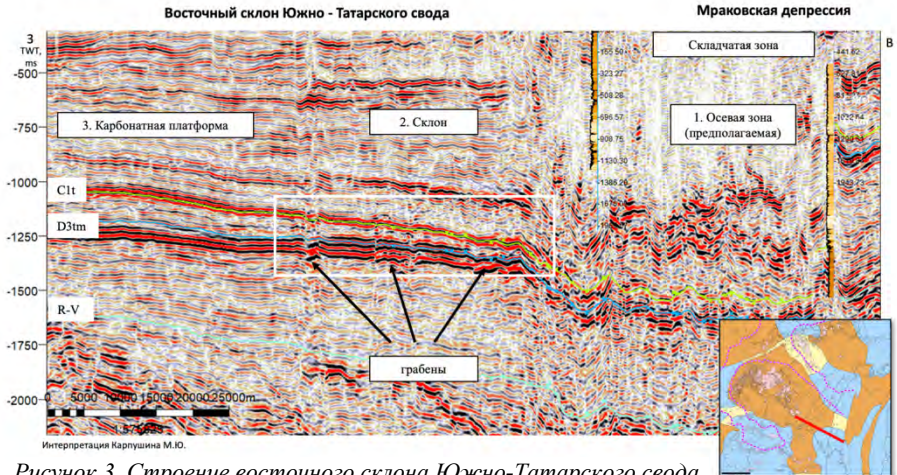
Рисунок 3. Стрoение восточного склона Южно-Татарского свода
