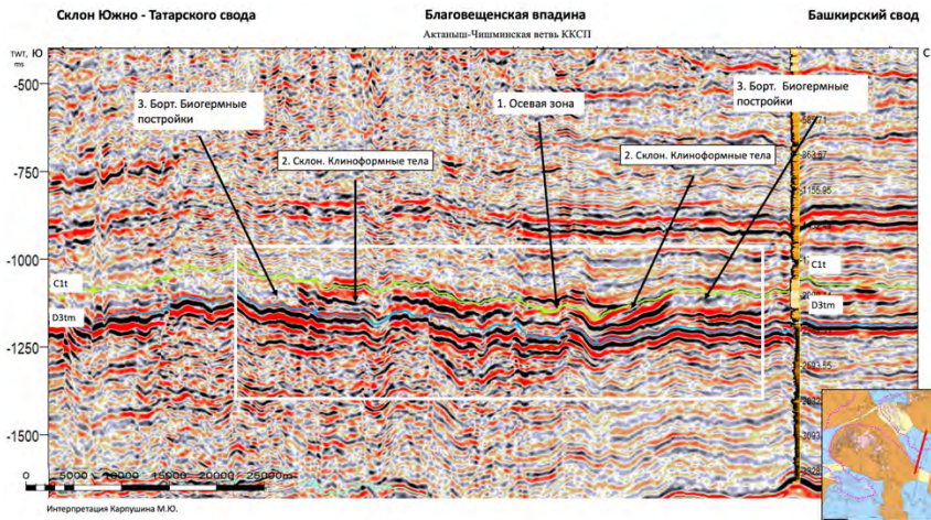
Рисунок 2. Выделение сейсмо-фациальных зон в разрезе франко-турнейского ССК. Сейсмический разрез проходит вкост простирания Камско-Кинельской системы прогибов.
