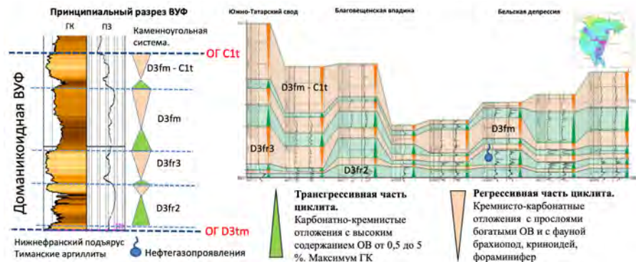
Рисунок 5. Циклиты и их лито-стратиграфическая корреляция в разрезе доманикоидного франско-турнейского комплекса отложений.
