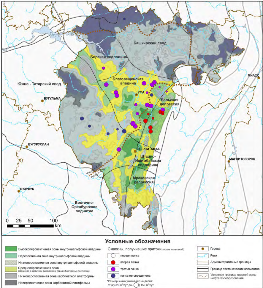
Рисунок 10. Перспективы нефтегазоносности доманикоидного среднефранско-турнейского комплекса.
