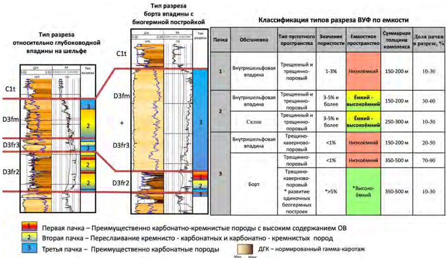
Рисунок 9. Распределение нетрадиционных природных резервуаров доманикоидного типа в разрезе и их связь с фациально-палеогеографическими зонами формирования высокоуглеродистой толщи.
