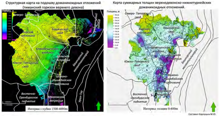
Рисунок 4. Структурная карта (слева) тиманского горизонта и суммарная карта толщин (справа) верхнефранско-нижнетурнейских доманикоидных отложений
