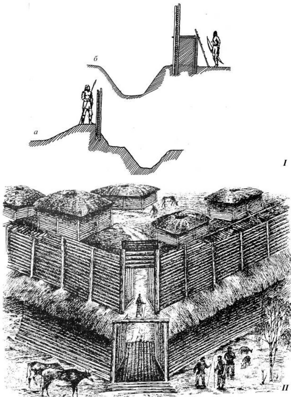
Рис. 121. Рафайловское городище. Реконструкции. I - однорядная защитная стена (a); двухрядная с забутовкой и настилом для стрелковой галереи (б); II - крепость раннего этапа [по Матвеева и др., 2005. Рис. 68, 69].
