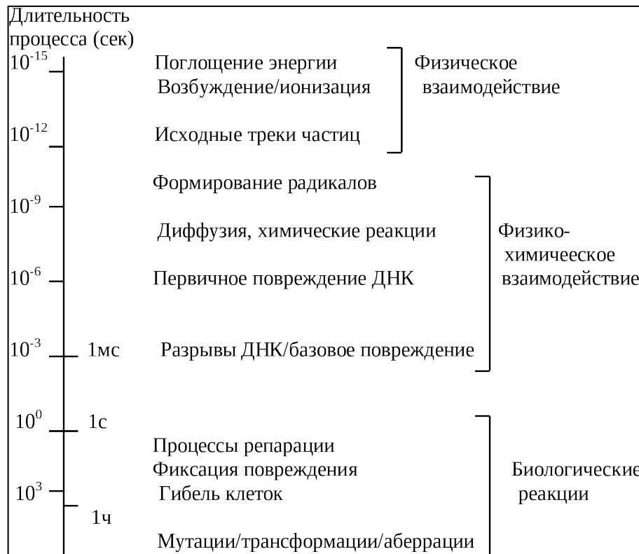
Рисунок 1.11 – Временной масштаб процессов, происходящих в биологических системах при их облучении ионизирующим излучением (процессы разделены на стадии) [74].
